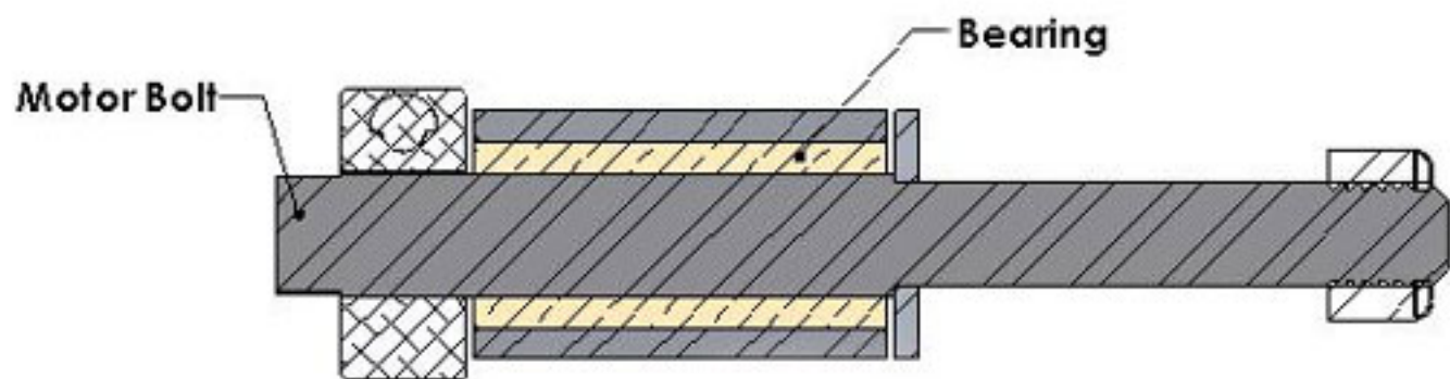
SECTION A-A
